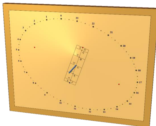
Orologio solare analemmatico vertical declinante verso Est (20° est)
