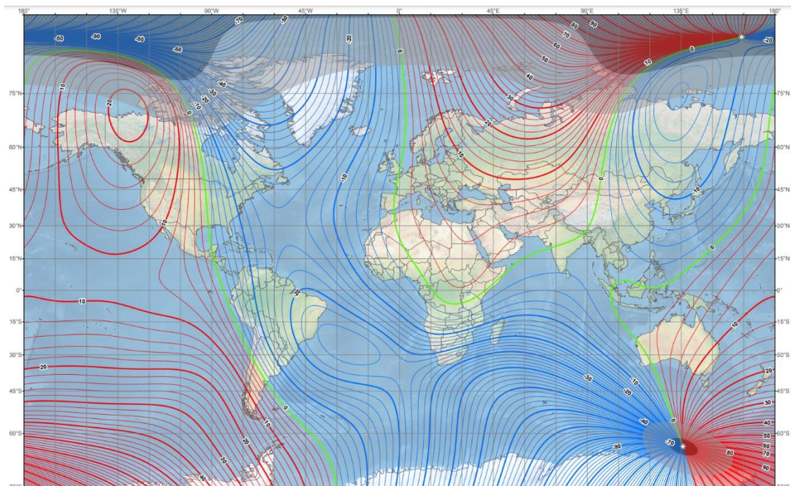
Declinazione magnetica, epoch 2020
