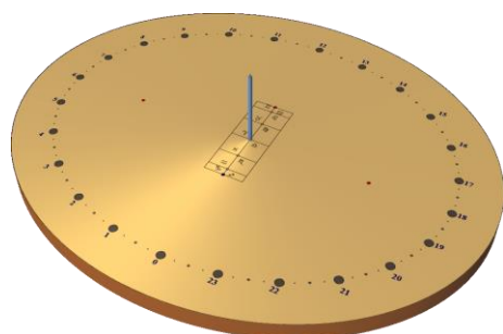
Orologio solare analematico orizzontale calcolato per Berlino, Germania (52° 30' N)
