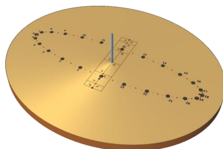
Orologio solare analematico orizzontale calcolato per Bangkok, Thailandia (13° 45' N)
