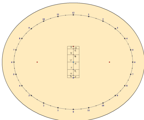
Cadran analemmatique horizontal pour Berlin, Allemagne (52° 30' N)
