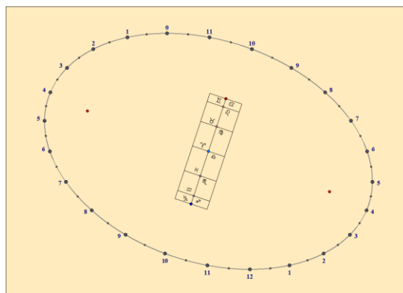
Cadran analemmatique vertical déclinant de 20^\circ vers l'Est
