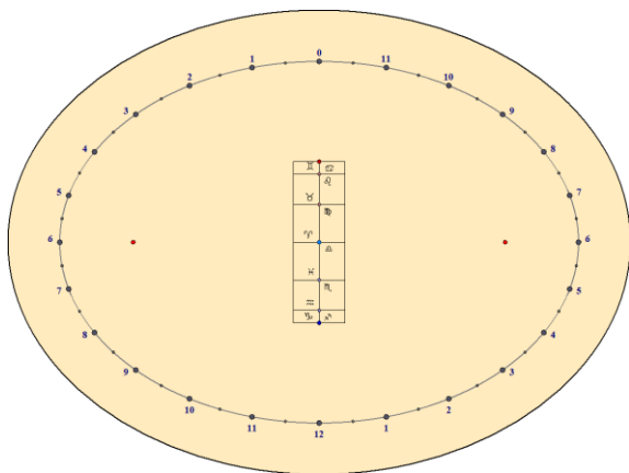
Cadran analemmatique vertical méridional
