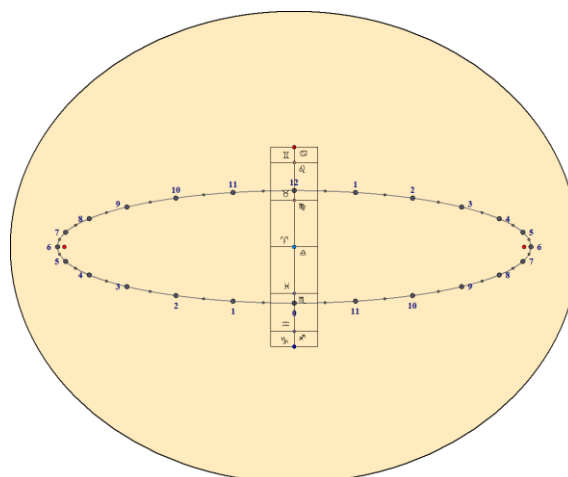
Cadran analemmatique horizontal pour Bangkok, Thaïlande (13° 45' N)
