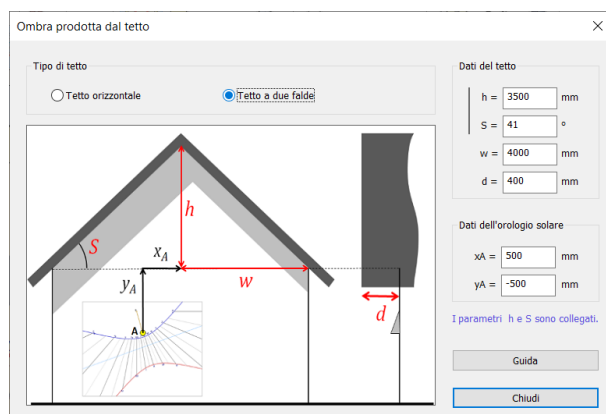
Configurazione di tetto a capanna
