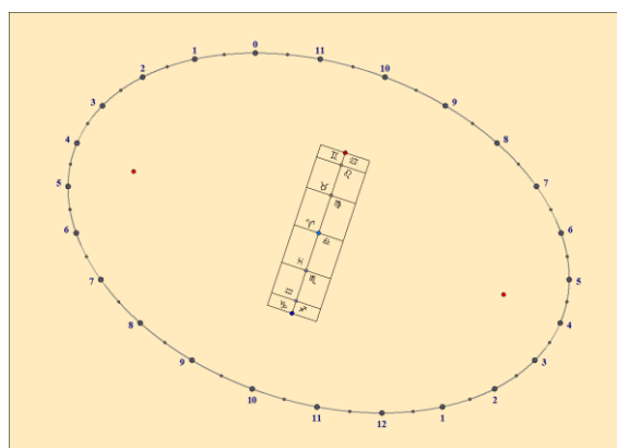
Orologio solare analemmatico vertical declinante verso Est (20° est)
