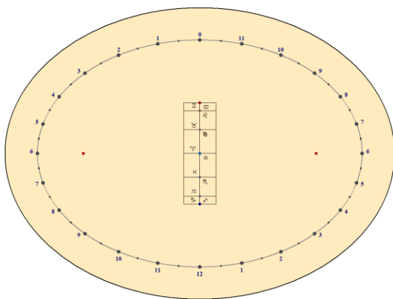
Orologio solare analemmatico vertical declinante verso Sud
