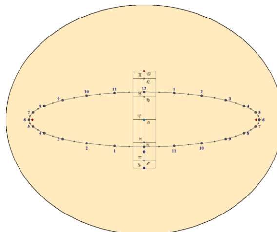
Orologio solare analemmatico orizzontale calcolato per Bangkok, Thailandia (13° 45' N)
