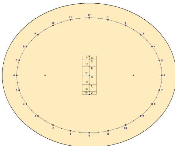
Orologio solare analemmatico orizzontale calcolato per Berlino, Germania (52° 30' N)
