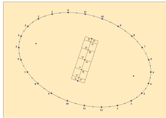
Vertikale abweichende analemmatische Sonnenuhr (20° Ost)
